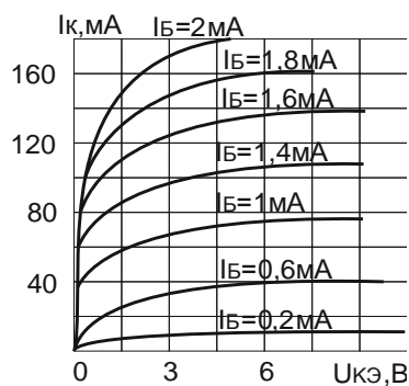
Входные характеристики КТ3107 А, В
