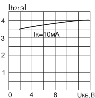
Зависимость модуля коэффициента передачи тока от напряжения коллектор-база
